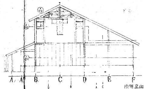
南側立面図
