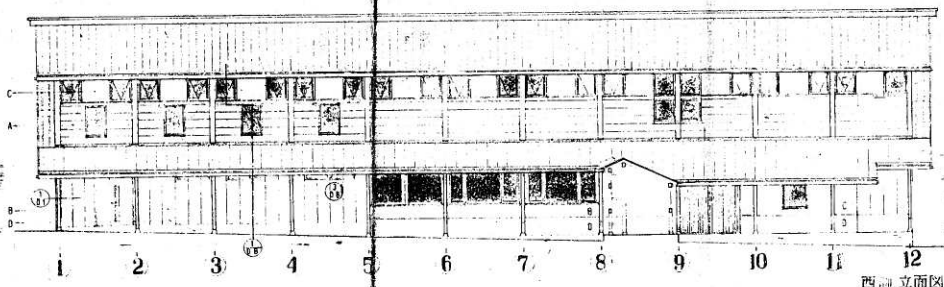
西側立面図
