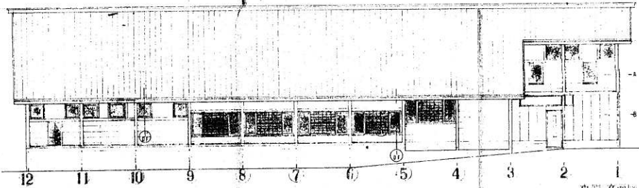
東側立面図
